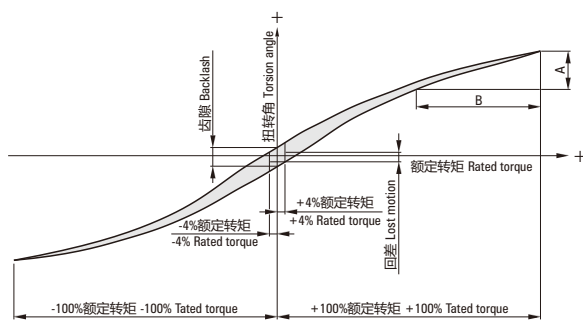
图1—迟滞曲线 Hysteresis curve
